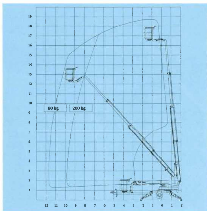
Arbejdsdiagram for trailermonteret lift.
